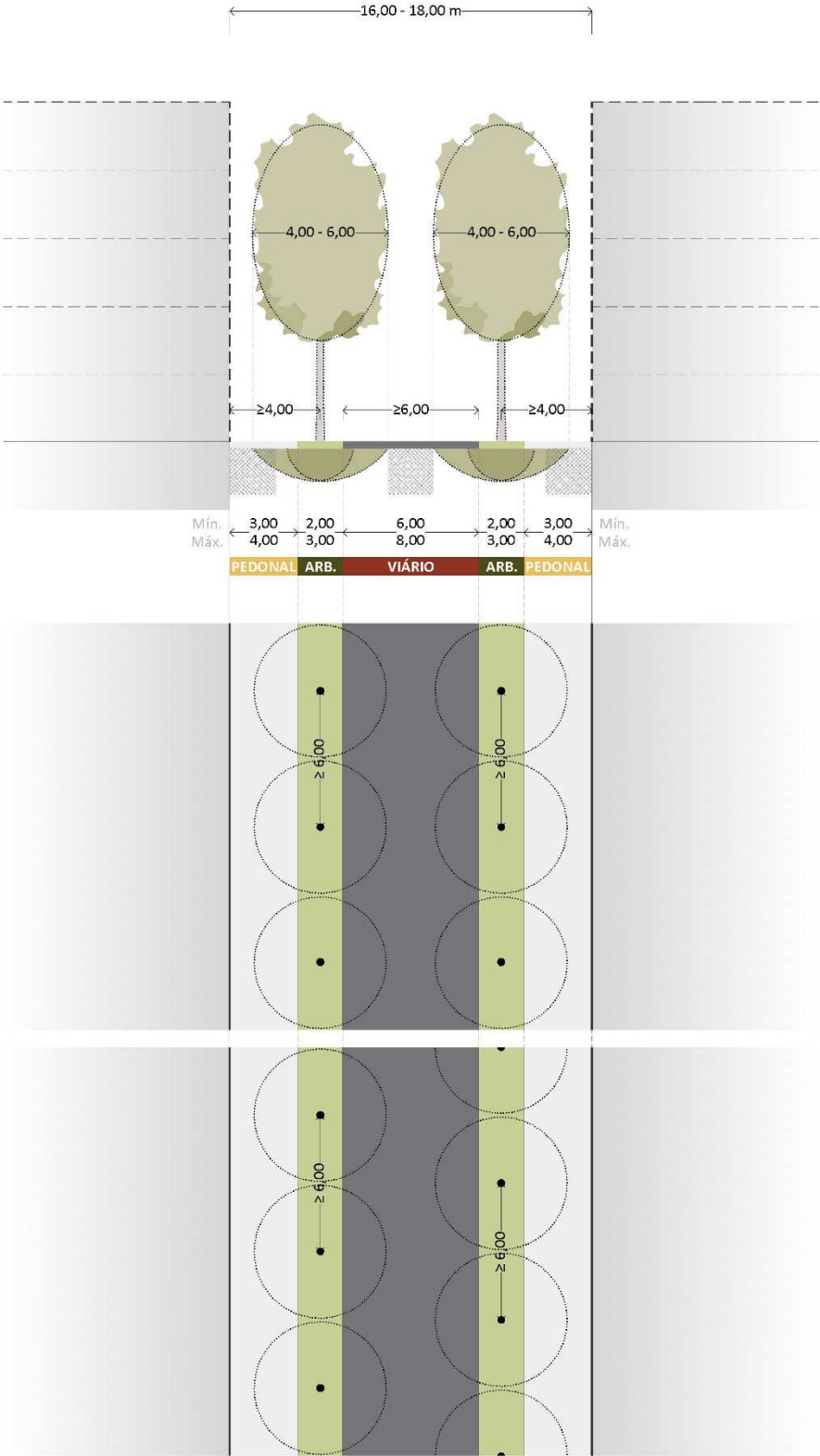
Figura 5.12 – Representação do modelo 4, em corte e em planta.
